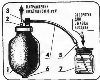
1 — резиновая груша, 2 — воздушный патруб- бок, 3 — конус с соплом, 4 — гибкий шланг, 5 — металлическая игла, 6 — воздушный клапан, 7 — баллончик для краски.
